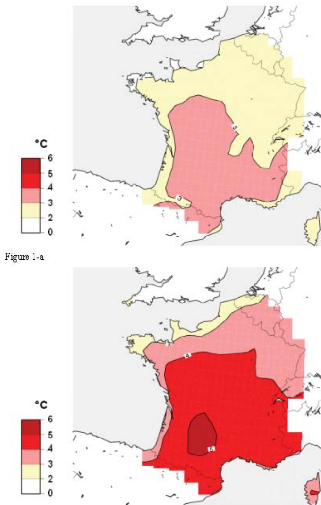
Figure 1 : Changements de températures moyennes d'été (mois de juin-juillet-août) simulés pour la période 2070-2099 par rapport à la période 1960-1989, suivant les scénarios B2 (a) et A2 (b). (Source IMFREX, 2004)
